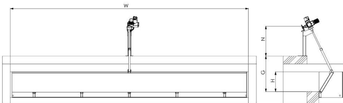
Wymiary zastawki w mm
