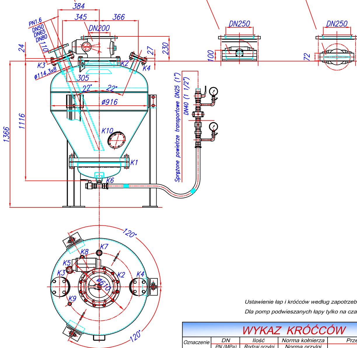
ZAMKNIĘCIE DZWONOWE ZD-200/250 EES-3-01-01
